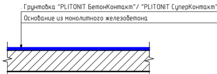
Рис.12. Конструктивный разрез №1.
